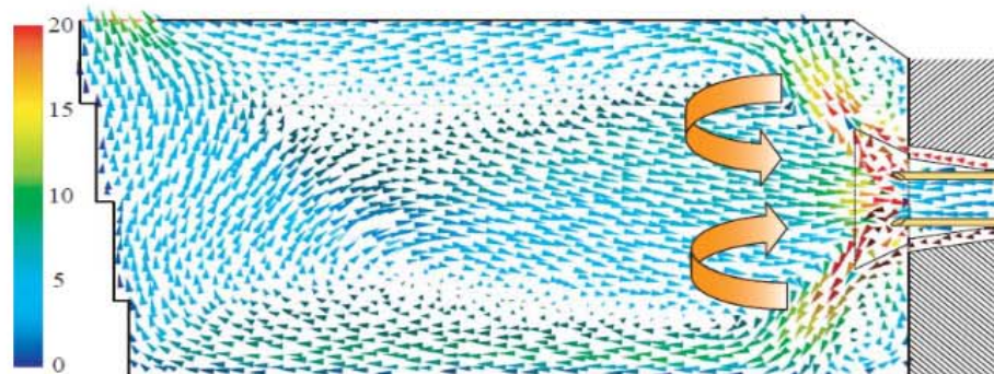
流速分布 [m/s]
