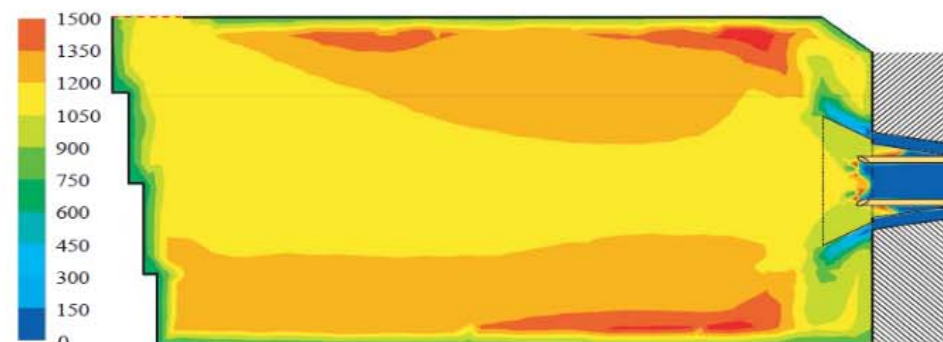
温度分布 [°C]
