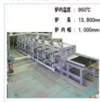
高張力鋼板連続加熱炉
